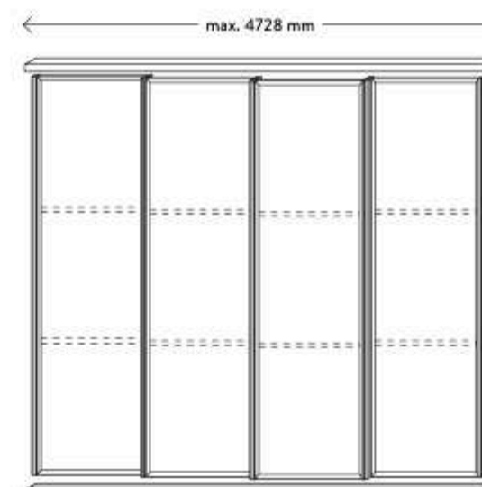
GSSET-010 3-läufiges Gleittürsystem mit 4 Türen
